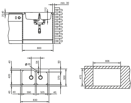
Instalación en encastre
