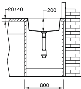
Instalación en encastre
