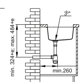
Huevo bajo encimera
