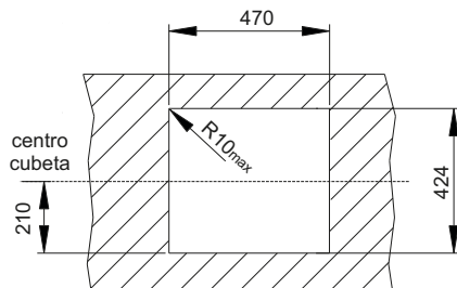
Hueco encastre
