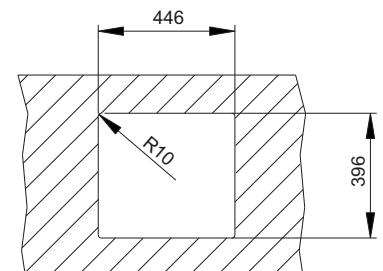
Hueco Bajo Encimera
