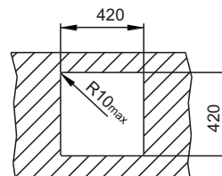
Huevo de encastre
