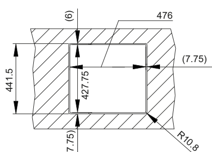
Hueco enrasado
