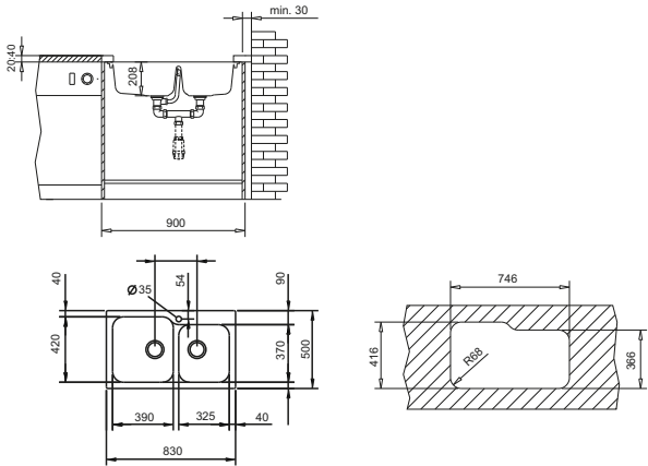
Instalación bajo encimera
