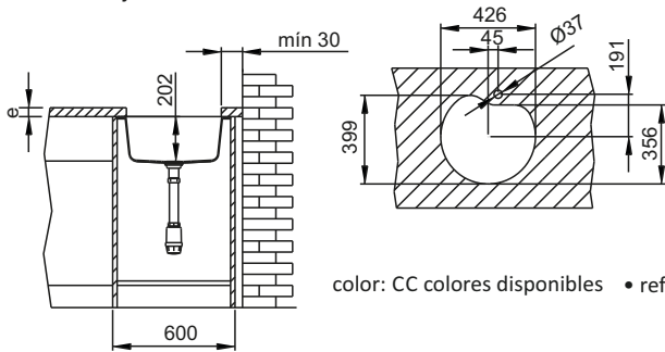
Instalación bajo encimera
