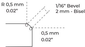
STANDARD EASED EDGE CANTO SENCILLO Only for squares and rectangles Solo en cuadrados y rectángulos
