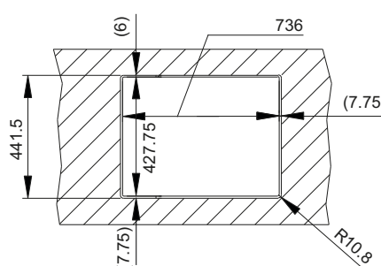
Hueco enrasado
