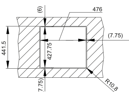
Hueco enrasado
