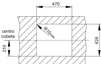
Hueco encastre
