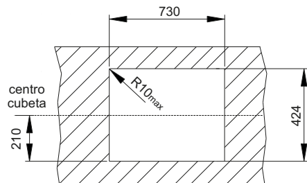
Hueco encastre
