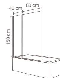
Mampara bañera RS-100 + RS-110 transparente (medida total 126 cm)
